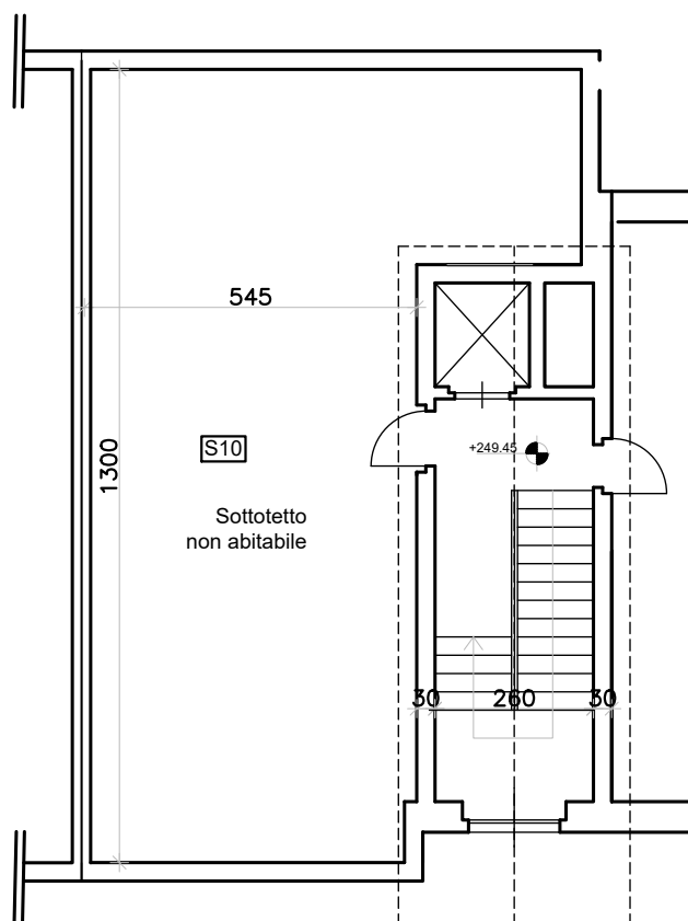
PIANTA PIANO SOTTOTETTO - ED. CONV.
